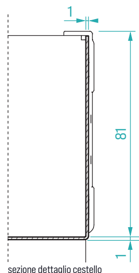
sezione dettaglio cestello
