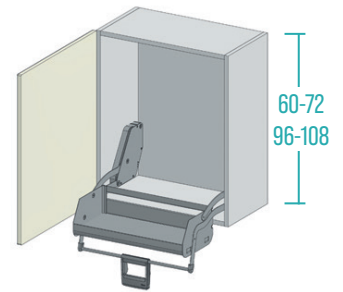
Pensile/Wall unit/Élément haut Mueble alto/подвесного шкафчика
