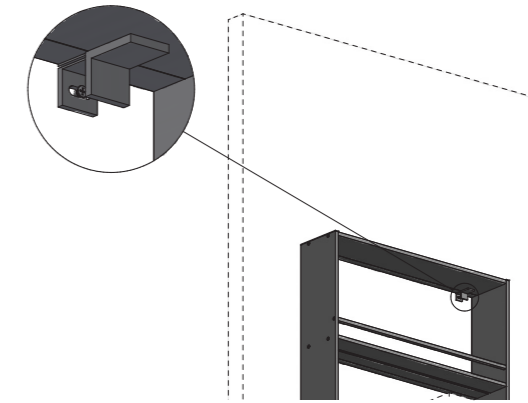
Particolare fissaggio a muro Wall fixing detail
