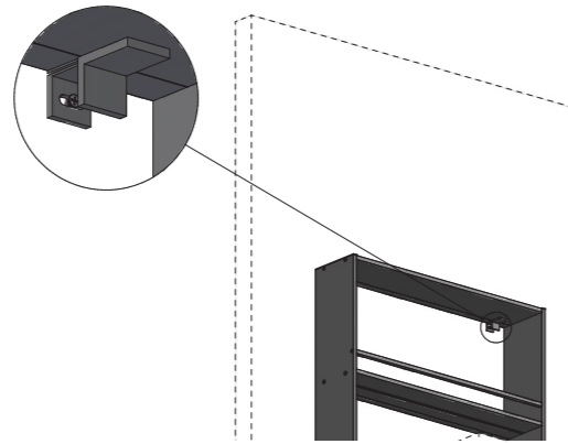
Particolare fissaggio a muro Wall fixing detail
