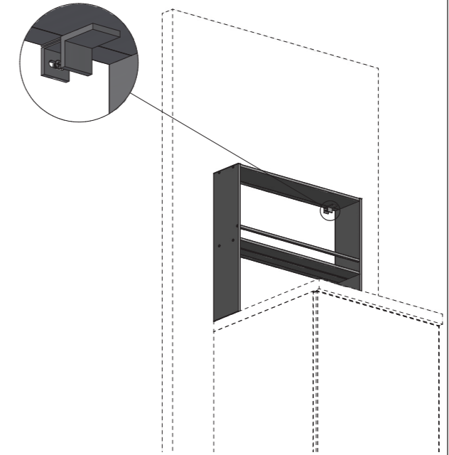
Particolare fissaggio a muro Wall fixing detail
