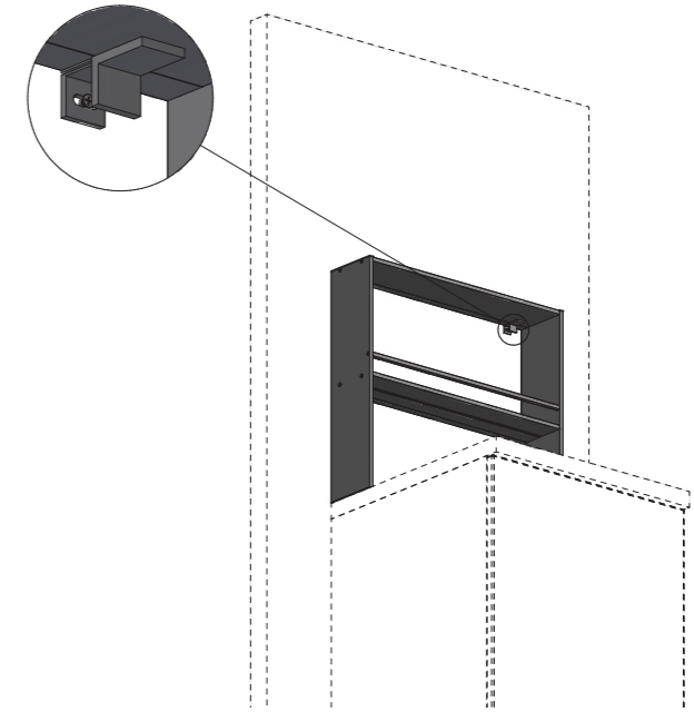
Particolare fissaggio a muro Wall fixing detail
