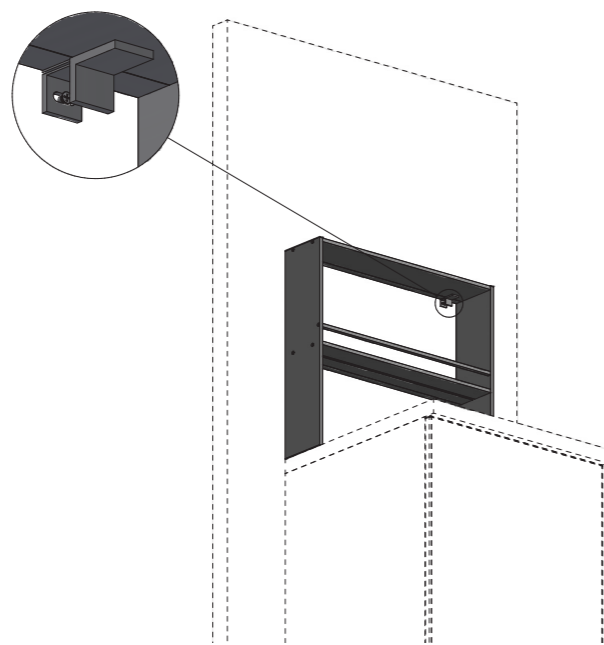
Particolare fissaggio a muro Wall fixing detail
