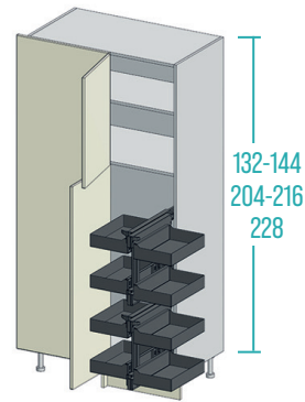
Colonna angolo/Corner column Colonne d'angle/Columna angulares Угловые шкафы-пенала
