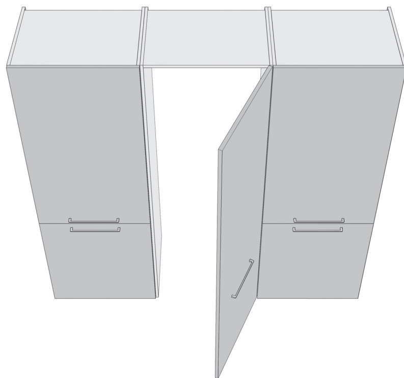
COMPOSIZIONE CON SISTEMA "PASS", VERSIONE "PULL-OUT", ANTA FINO A TERRA COMPOSITION WITH "PASS" SYSTEM, "PULL-OUT" VERSION, DOOR DOWN TO GROUND
