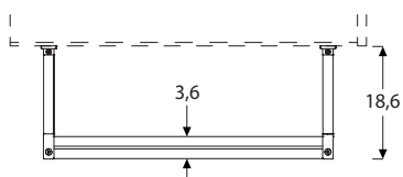
VISTA SUPERIORE TOP VIEW
